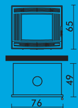
PELLBOX (funzionamento a pellet)
